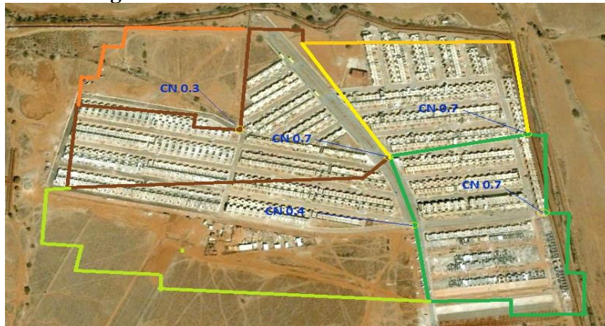
Figura 1.4 Subcuencas delimitadas con WMS
