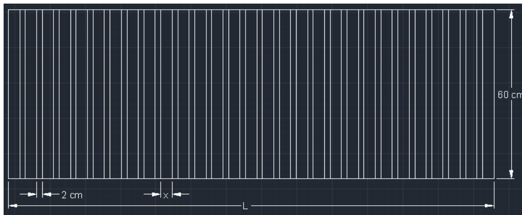
Figura 1.6 Dimensiones de las bocas de tormenta
