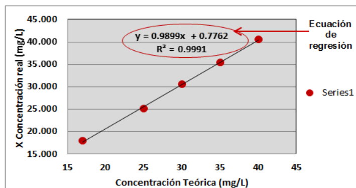
Gráfico 10 Curva de calibración para determinar el límite de cuantificación de los SST
