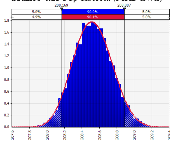
Gráfico 4.13 Fdp discreta (MRD kWh)
