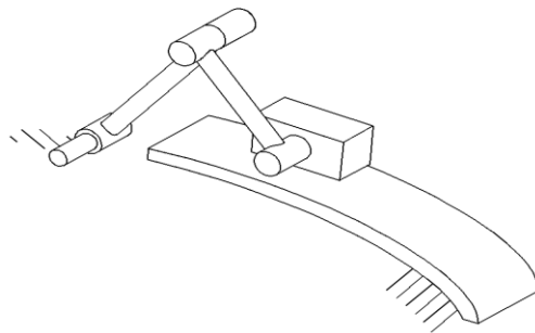
Figura 18.3 Mecanismo diseñado para generar la función \theta = \phi^{0.3} y seguir una trayectoria elíptica
